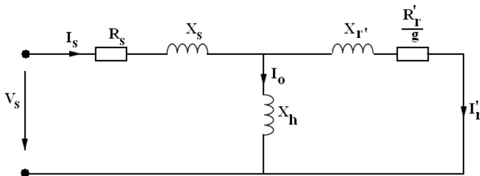
Figure4. 4.Schéma équivalent simplifié de la machine asynchrone
