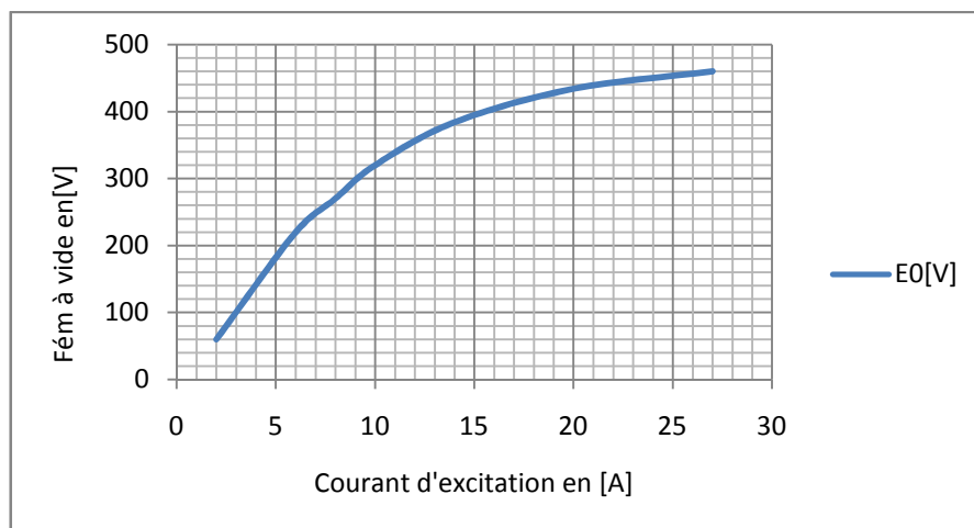
Fig.7 f.é.m. en fonction de I_{ex}
