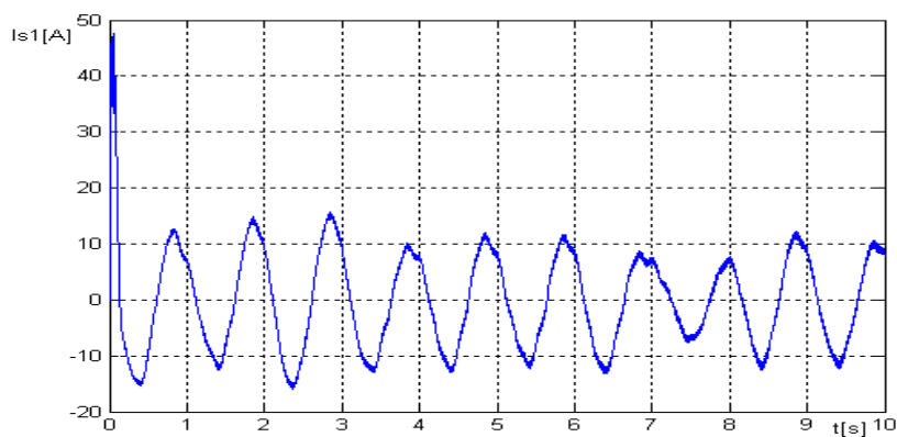
Figure4. 27.Courant statorique en fonction du temps
