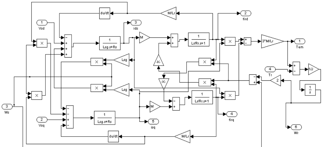
Figure4. 10.Schéma de la machine asynchrone sous Simulink
