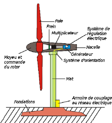
Figure1. 4.Eléments constitutifs d'une éolienne
