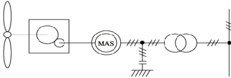
Figure4. 1.Système éolien utilisant la génératrice asynchrone à cage
