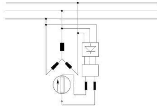
Figure 5.MS avec un système d'auto-excitation
