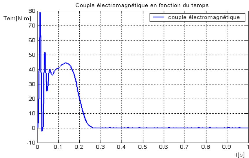
Figure4. 15.Couple électromagnétique en fonction du temps
