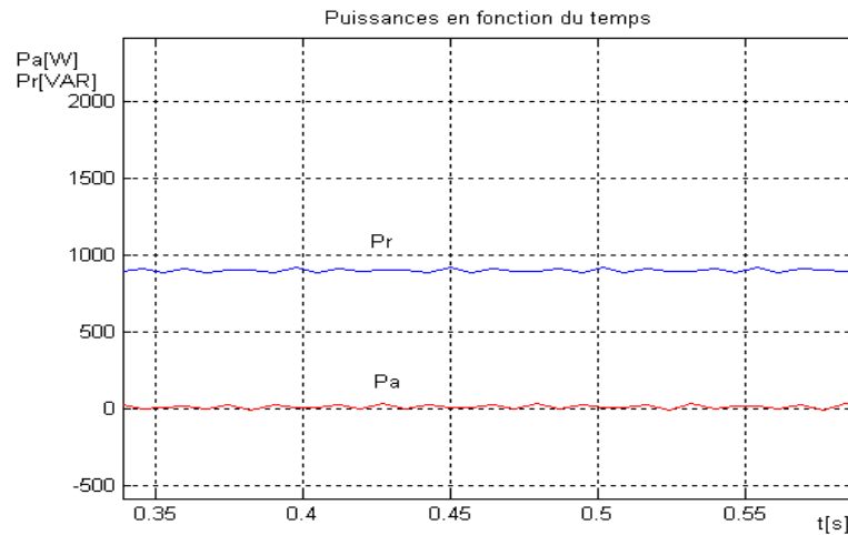
Figure4. 20. Vue agrandie de la figure 4.19 à t = 0.6[s]
