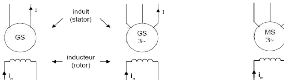
Figure 1. Symbole d'une machine synchrone
