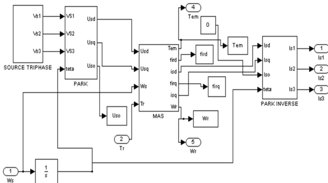
Figure4. 13.Schéma de simulation de la machine asynchrone
