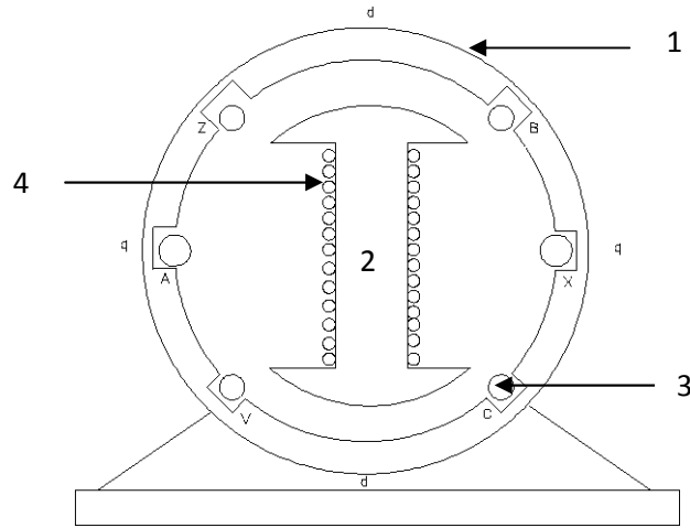
Figure 2. Coupe d'une machine synchrone
