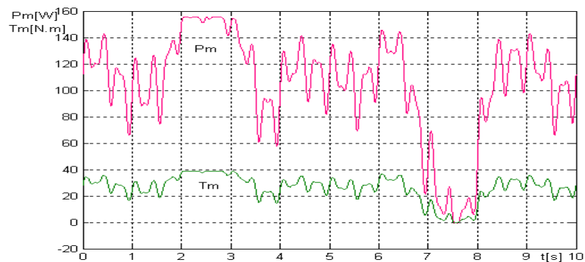
Figure4. 25.Puissance et couple mécaniques de la turbine
