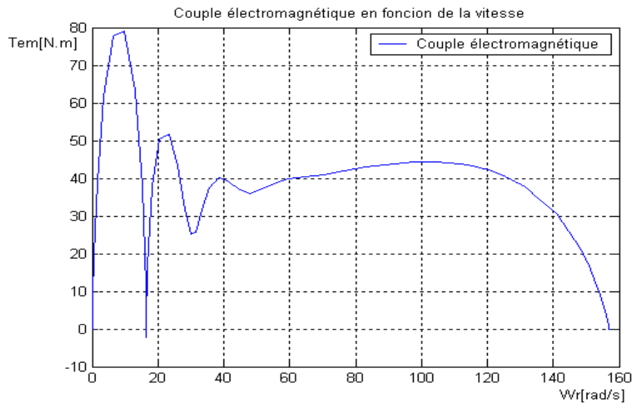
Figure4. 18.Couple électromagnétique en fonction de la vitesse rotorique
