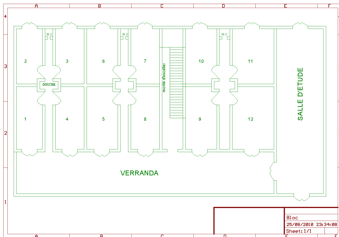
Figure2. 7.Schéma d'un appartement d'un bloc des étudiants
