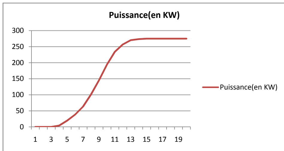
Figure2. 14.Courbe de puissance de l'aérogénérateur
