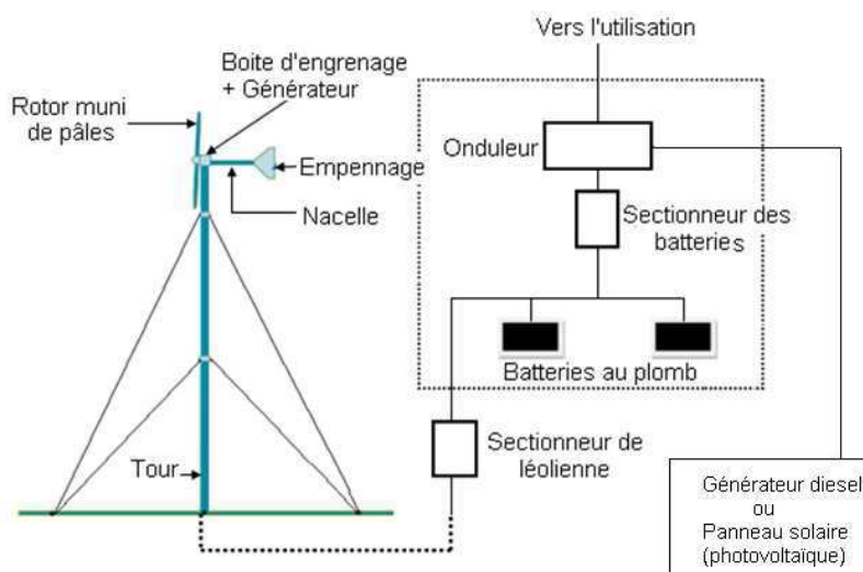
Figure1. 22.Composants d'un système éolien
