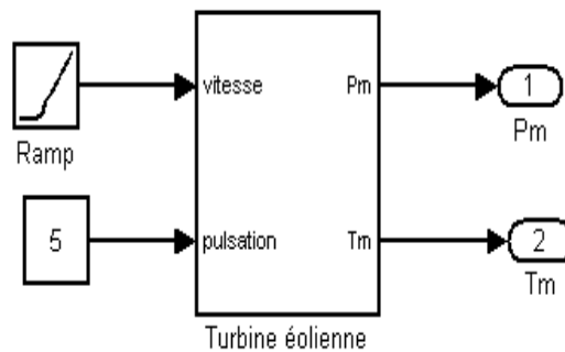
Figure4. 7.Schéma bloc de la turbine
