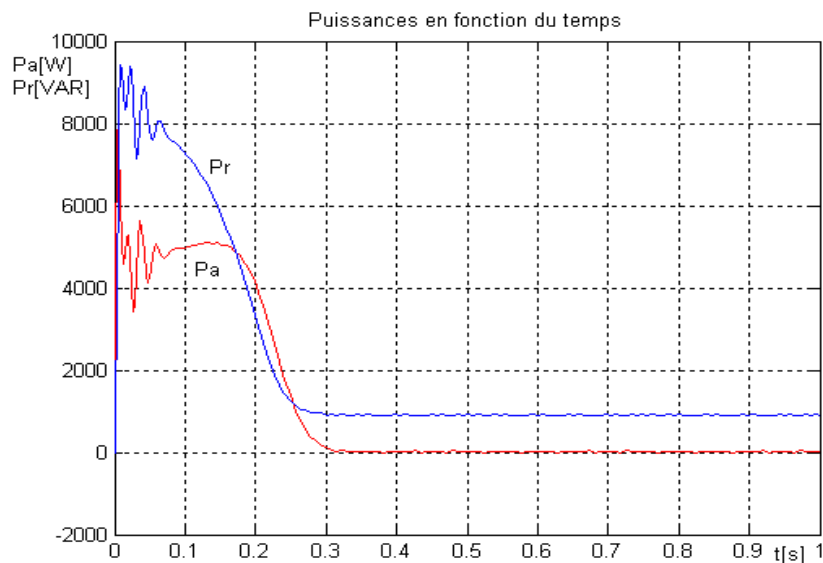
Figure4. 19.Puissances active et réactive en fonction du temps
