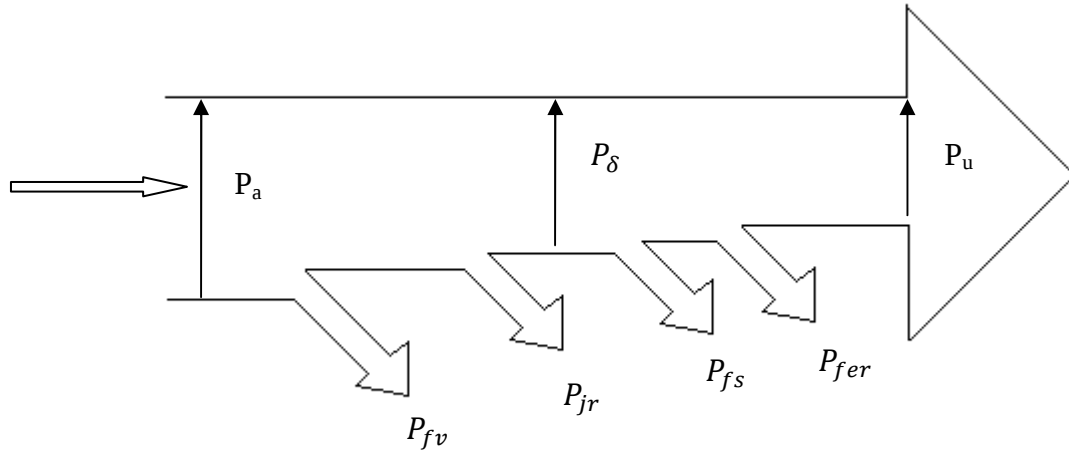
Figure.6 Bilan des puissances d'une MS
