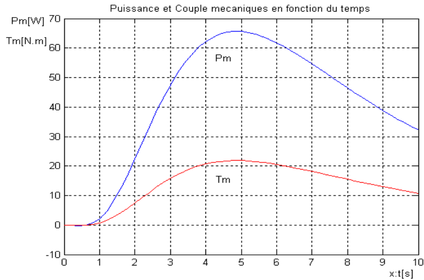
Figure4. 8.Puissance et couple mécanique de la turbine (pour \omega = 3[\text{rad/s}] )
