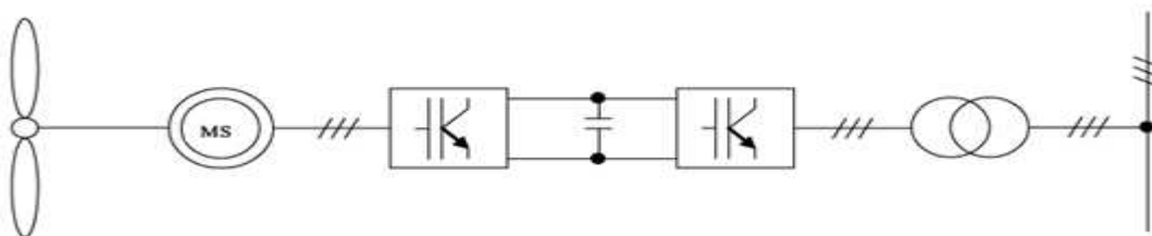
Figure1. 13.Système éolien basé sur la génératrice synchrone à aimants permanents
