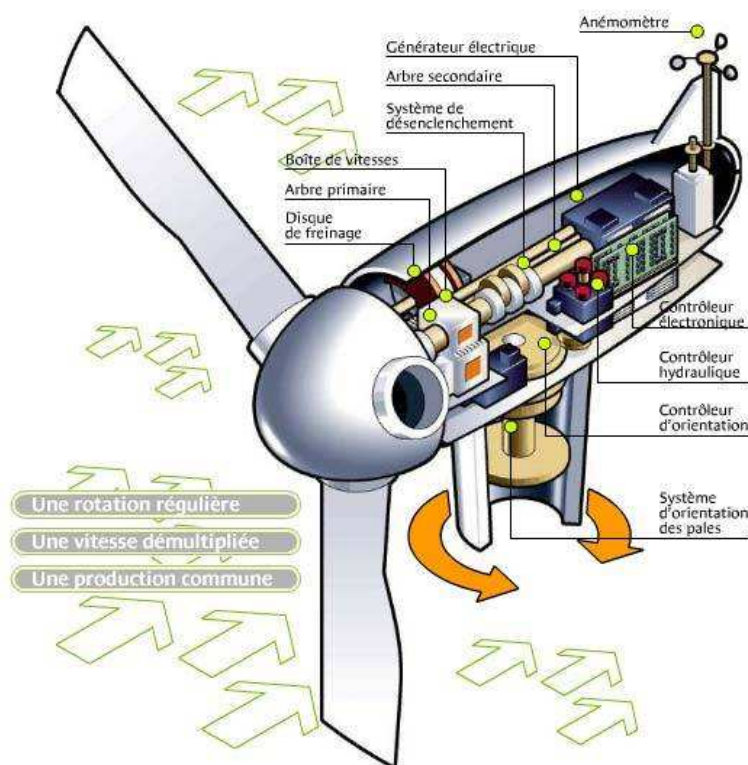
Figure1. 5.Vue éclatée d'une éolienne
