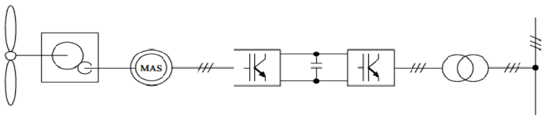
Figure1. 11.Système éolien basé sur la génératrice asynchrone à cage à fréquence variable
