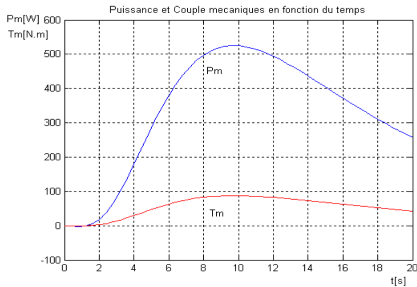
Figure4. 9.Puissance et couple mécanique de la turbine (pour \omega = 6[\text{rad/s}] )
