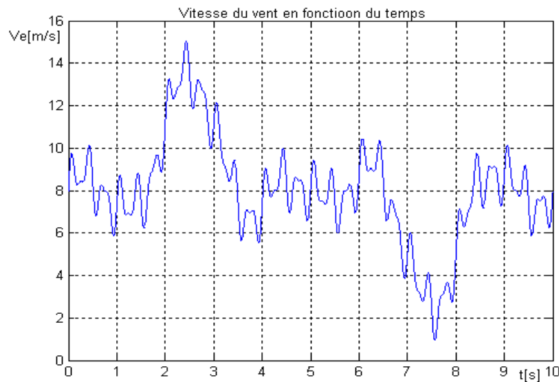
Figure4. 5.Courbe d'évolution de la vitesse du vent dans le temps.
