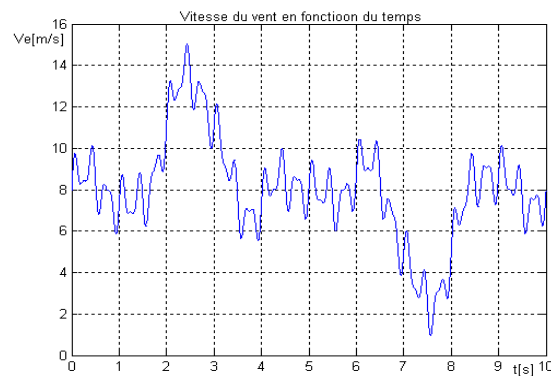
Figure4. 24.Courbe de variation de la vitesse du vent
