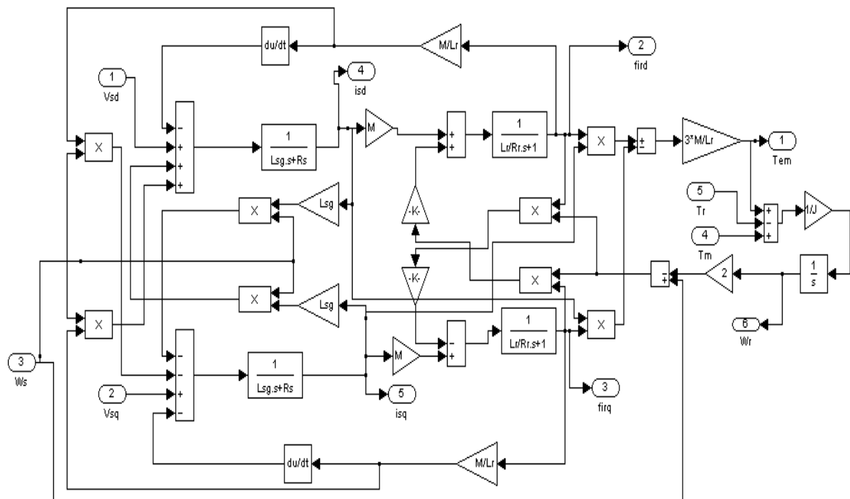
Comme nous le montre la figure 4.21, le bloc de machine asynchrone est modifié par l'existence d'un nouveau paramètre d'entrée, le couple mécanique de la turbine. La figure suivante donne la nouvelle structure du contenu de la machine.
