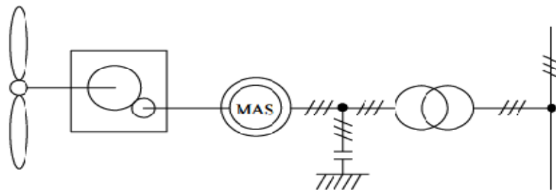
Figure1. 10.Système éolien utilisant la génératrice asynchrone à cage
