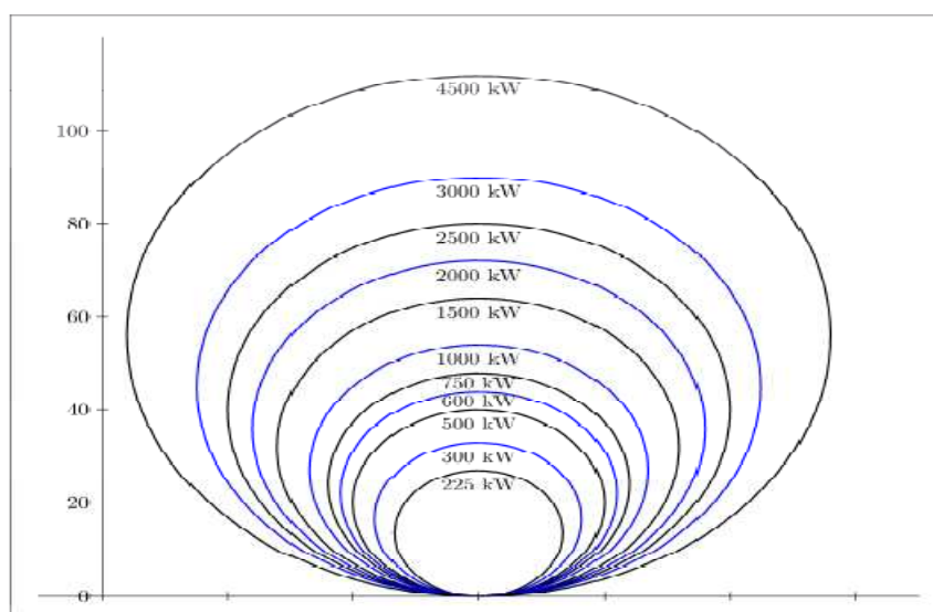
Figure1. 2.Taille des hélices en m et puissances en KW
