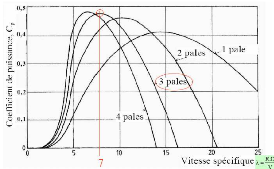
Figure4. 2.Coefficient de puissance en fonction de \lambda
