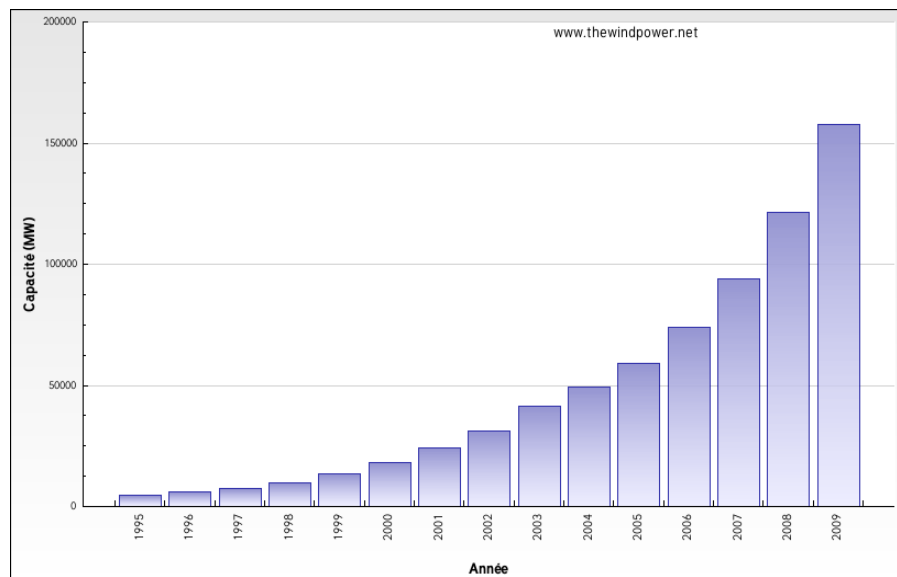
Figure1. 1.Evolution de puissances éoliennes installées dans le monde en MW
