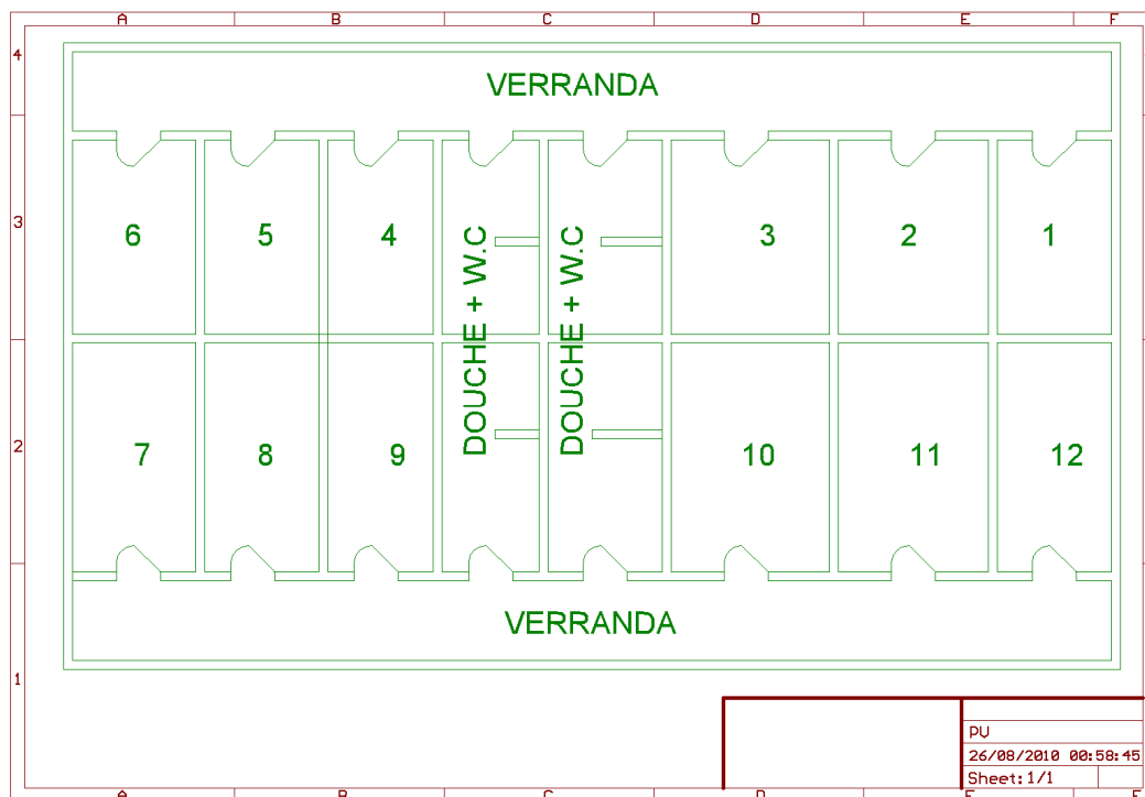
Figure2. 8.Schéma d'un appartement P.V des étudiants
