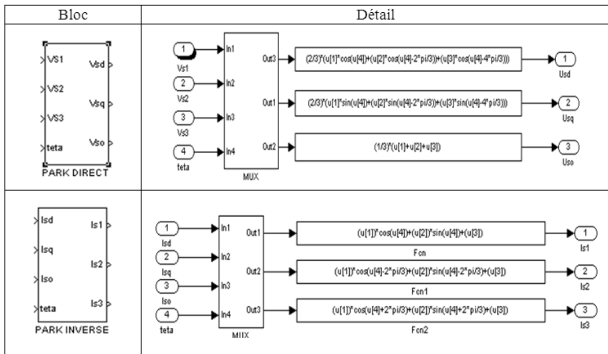
Figure4. 12.Blocs de transformation de Park
