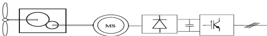
Figure1. 14.Système éolien utilisant la génératrice synchrone et un redresseur à diodes
