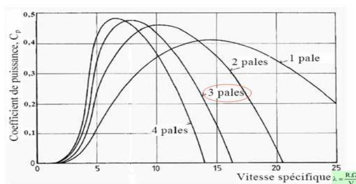
Figure1. 21.Abaque de choix du nombre de pales
