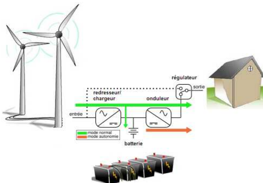
Figure2. 16.Système de production au complet
