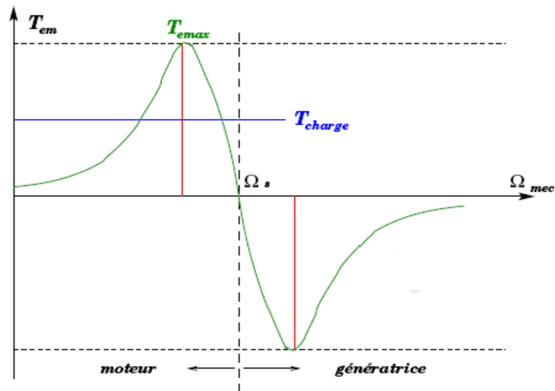
Figure4. 3.Caractéristique couple-vitesse d'une machine asynchrone
