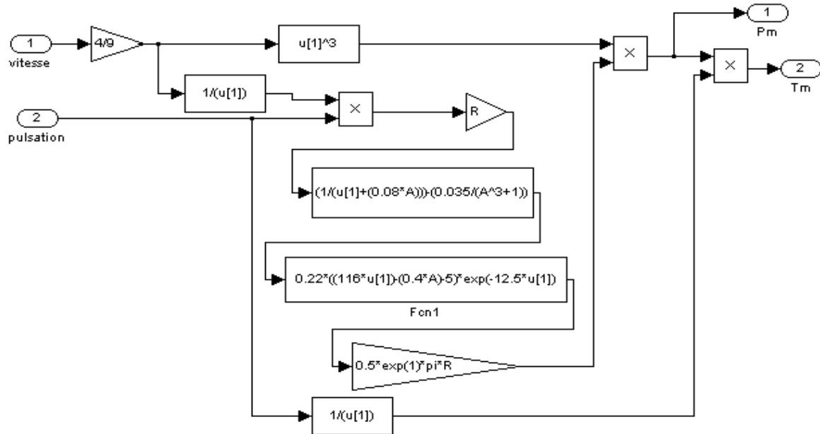
Figure4. 6.Modèle de la turbine sous simulink
