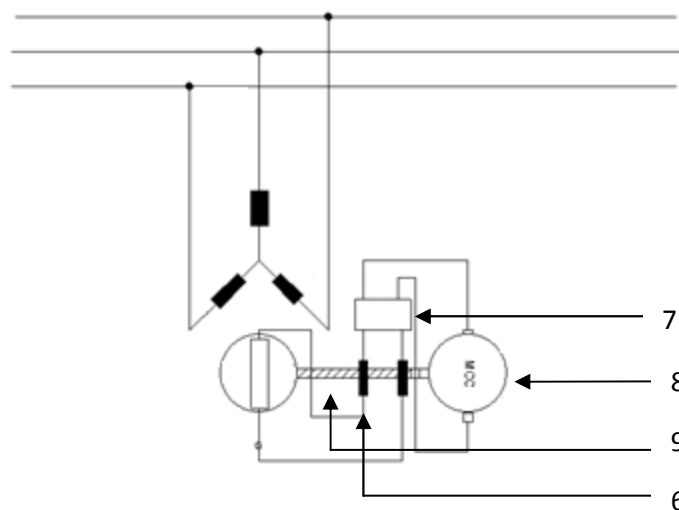
Figure 4. MS à excitation indépendante
