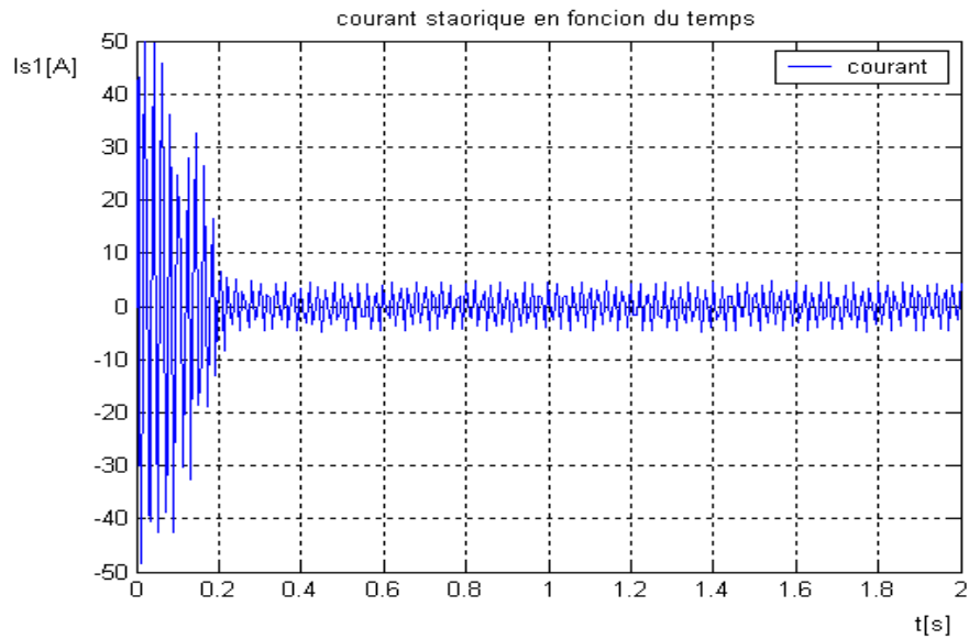
Figure4. 16.Courant statorique en fonction du temps
