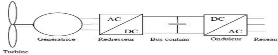
Figure1. 15.Système de production en général en petite puissance
