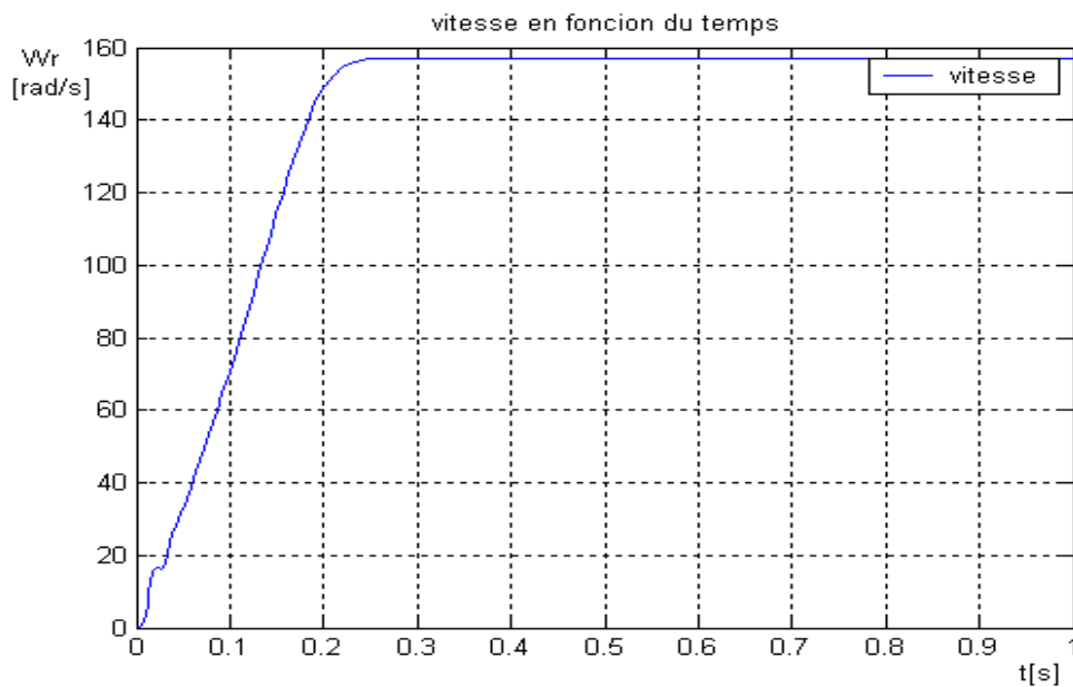
Figure4. 17.Vitesse du rotor en fonction du temps
