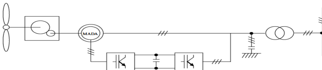
Figure1. 12.Système éolien à génératrice asynchrone à rotor bobiné
