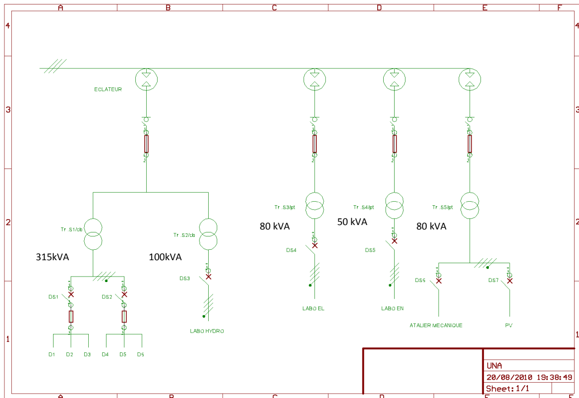
Figure2. 6. Schéma de distribution électrique de l'UNA
