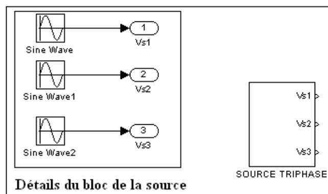
Figure4. 11.Schéma bloc de la source triphasée
