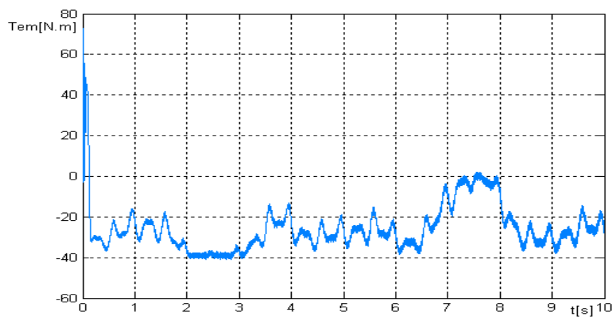
Figure4. 28.Couple électromagnétique en fonction du temps
