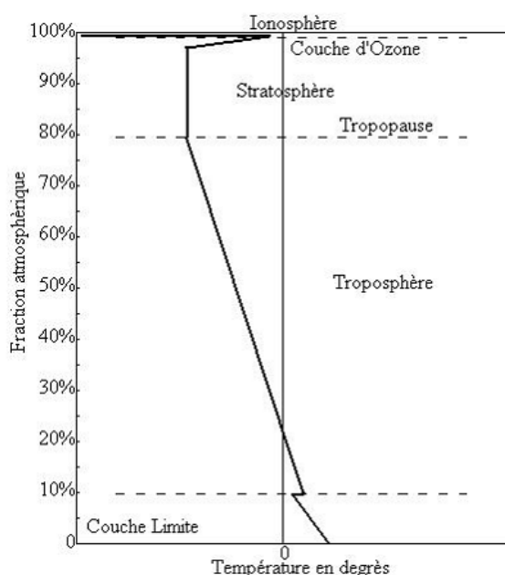
Figure2. 1.Vue schématique de la couche atmosphérique standard
