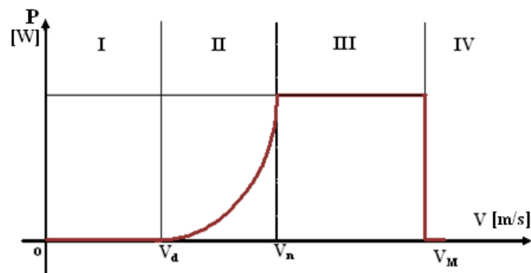
Figure1. 16.Caractéristique puissance-vitesse d'une éolienne
