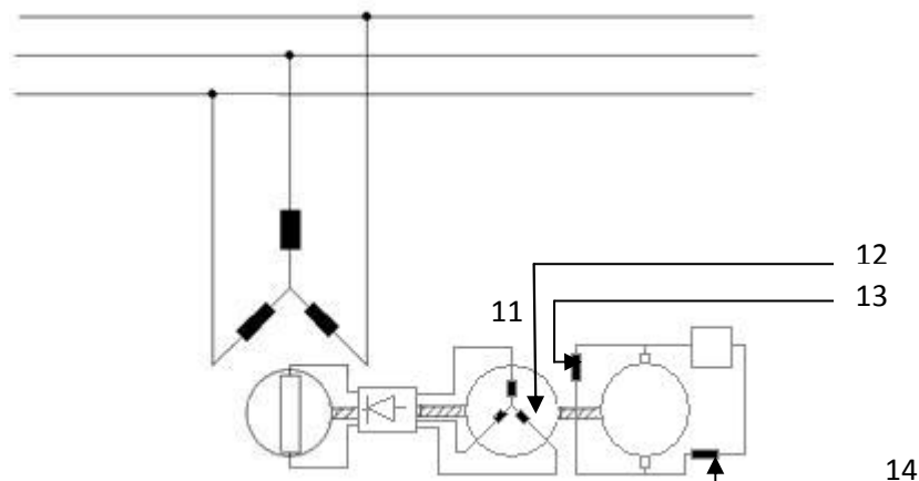
Figure 6.MS avec un système d'excitation sans contact
