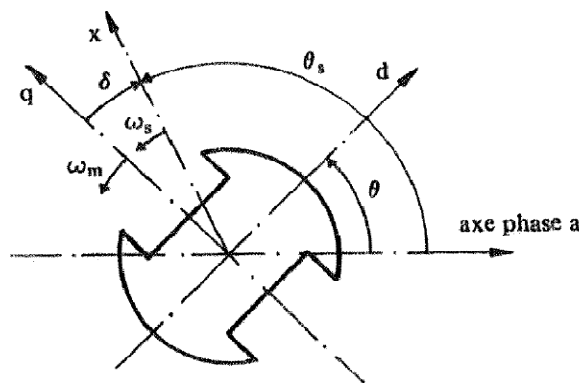
Figure. 6-4 Repérage des divers axes et angles [cf.1].
