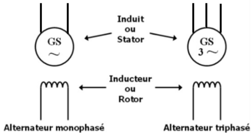
Figure. 3-3 : Alternateur monophasé et triphasé
