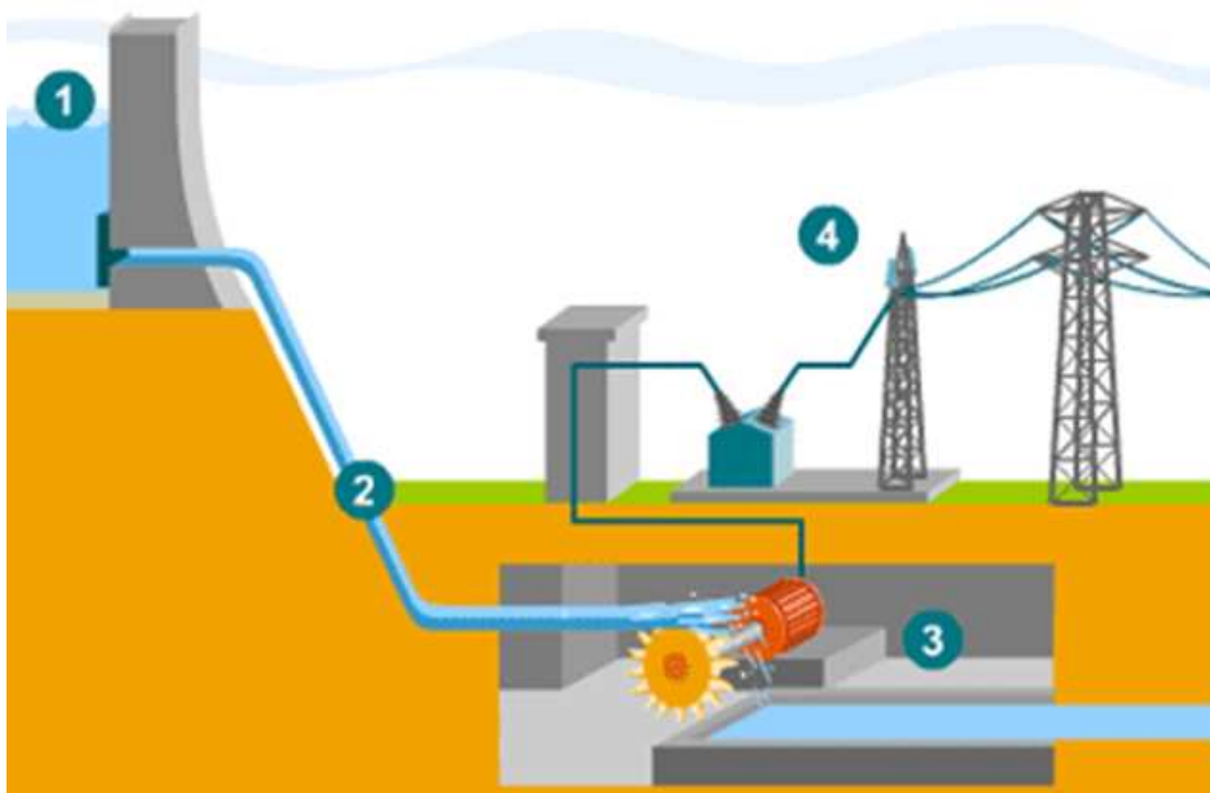
Figure. 1- 1 : Vue d'ensemble d'une microcentrale hydraulique
