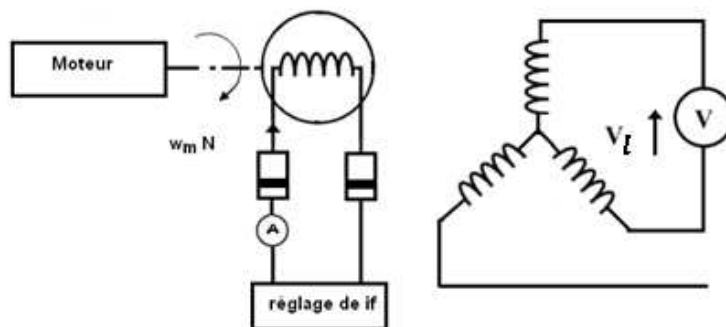
Figure 4-8 : Schéma équivalent à un enroulement d'une génératrice synchrone
