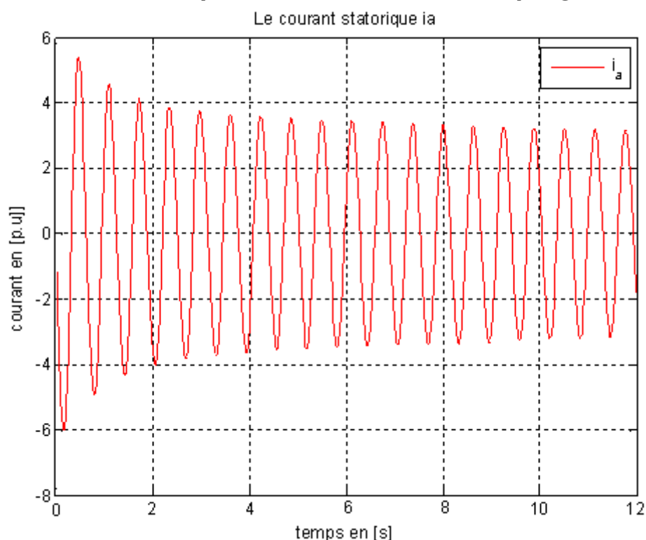
Figure : 7-1 Courant de phase statorique i_a .
