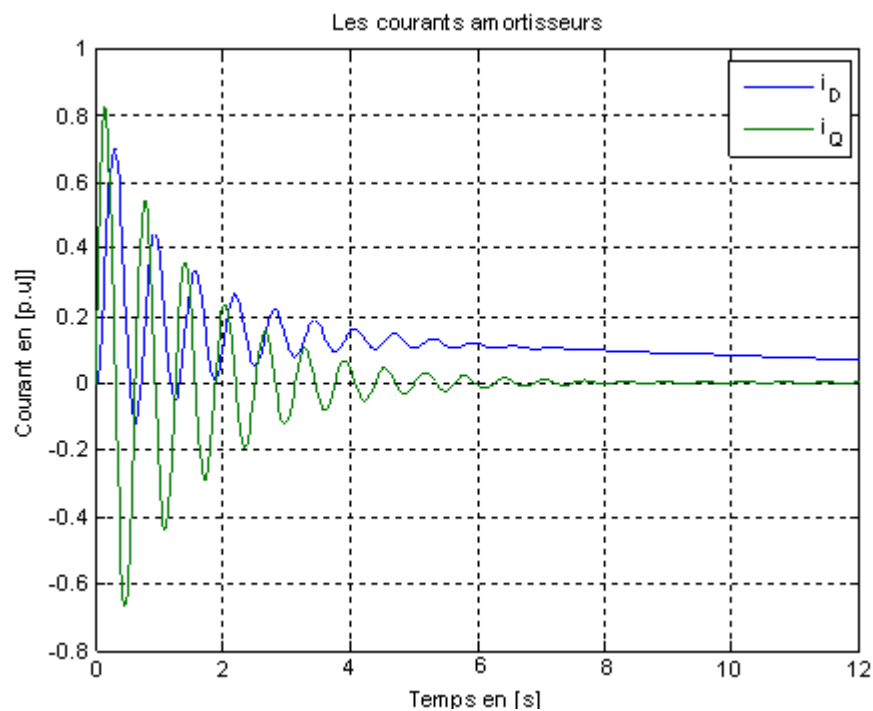
Figure : 7- 8 les Courants d'amortissements i_D et i_Q .
