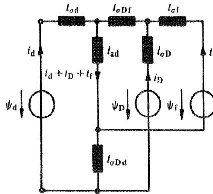
Figure 6-1 : Schéma équivalent pour les flux dans l'axe direct.
