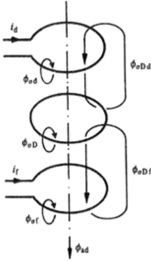
Figure 5-3 : Flux dans l'axe direct.
