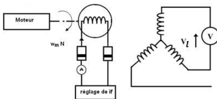
Figure 4-7 : Schéma équivalent à un enroulement d'une génératrice synchrone.
