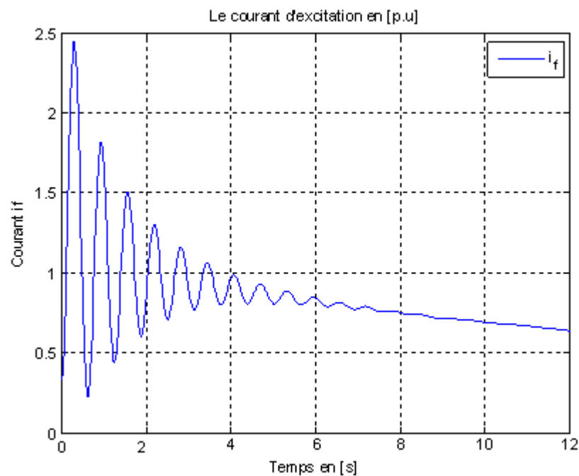
Figure : 7- 5 Courant d'excitation i_f .
