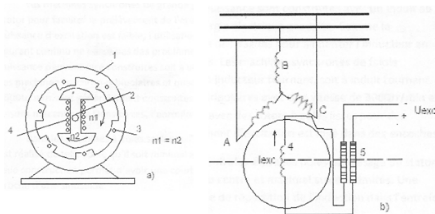
Figure. 3-7 : Principe de fonctionnement
