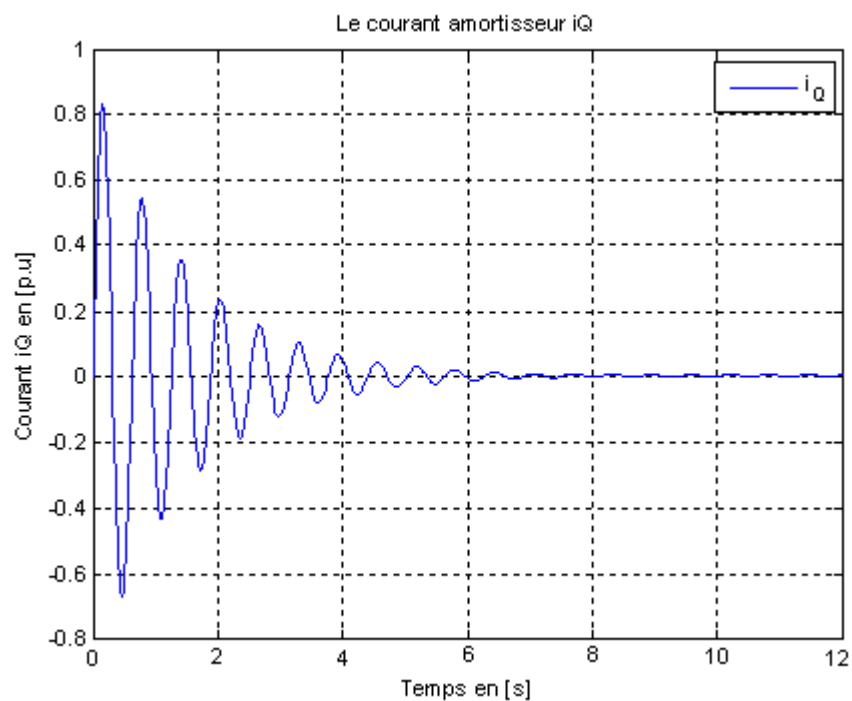
Figure : 7-7 Courant d'amortissement i_Q .
