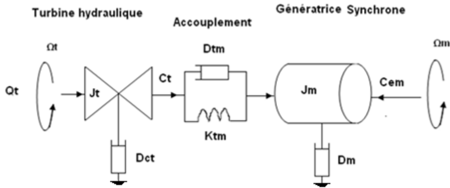
Figure 6-5 : couplage mécanique entre de la turbine hydraulique et la machine synchrone [cf.1].
