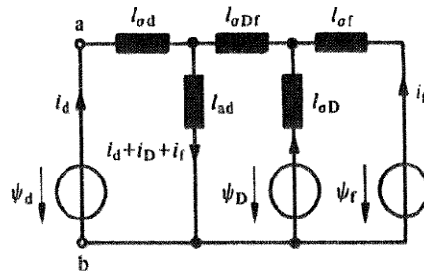
Figure 6-1 : Schéma équivalent pour les flux dans l'axe direct.
