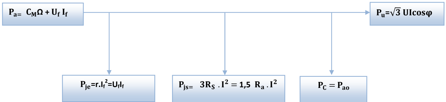
Figure.4-3 : Bilan des puissances
