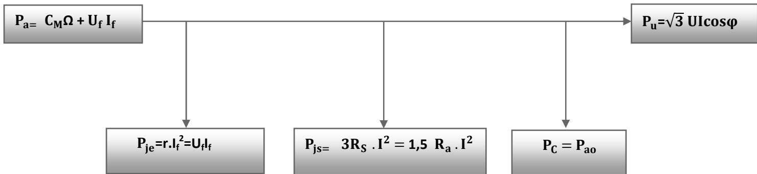
Figure 4-4 Bilan énergétique d'un alternateur synchrone
