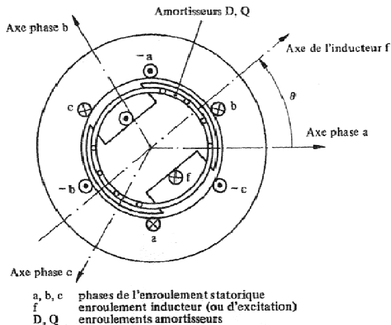
Figure.4-4 : Les différents enroulements d'une machine synchrone
