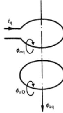
Figure 5 - 4 : Flux dans l'axe transversal [cf.1].
