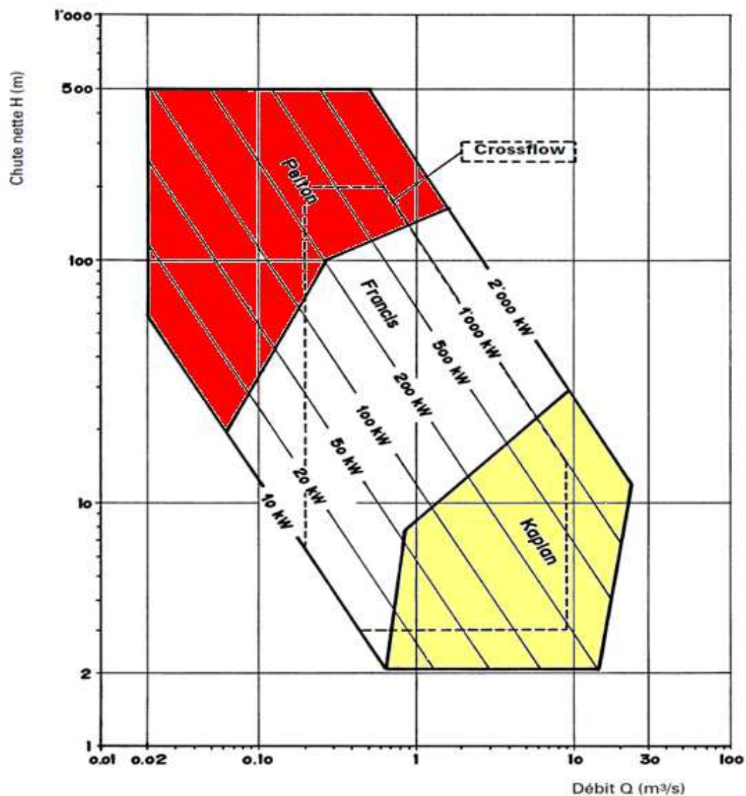
Figure.3-1 : Domaine d'utilisation des différents types de turbines (chutes nettes, débits, puissances) [Cf.8].
