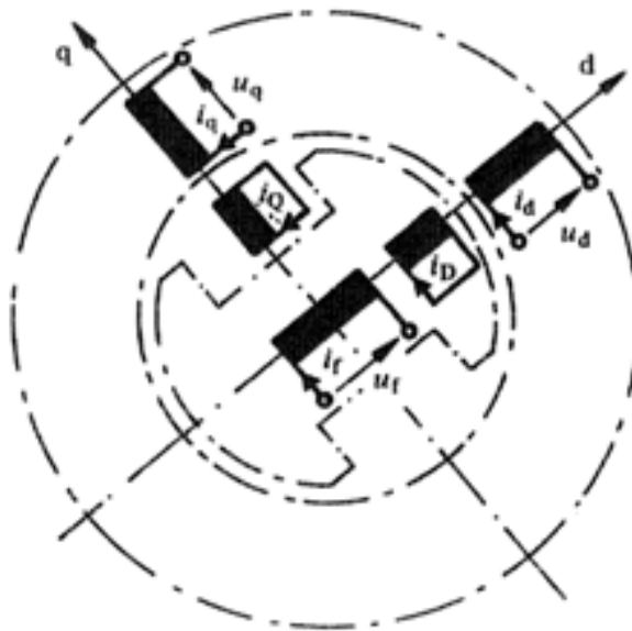
Figure.5-2 : Modèle de Park de la machine synchrone
