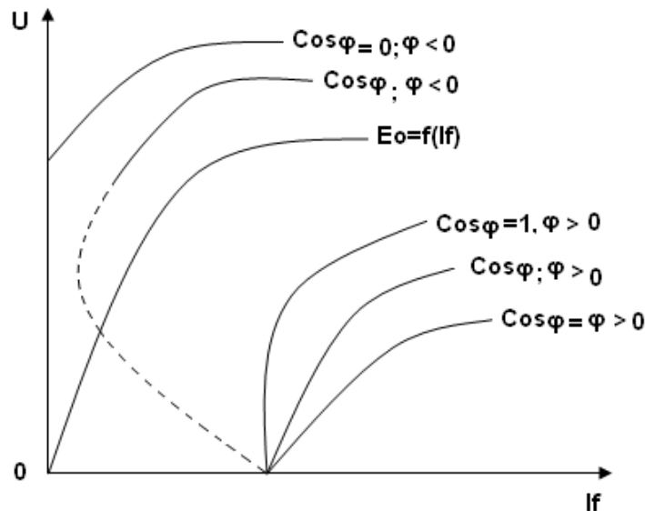
Figure .4-2 : Caractéristiques en charge d'un alternateur synchrone réaction d'induit :
