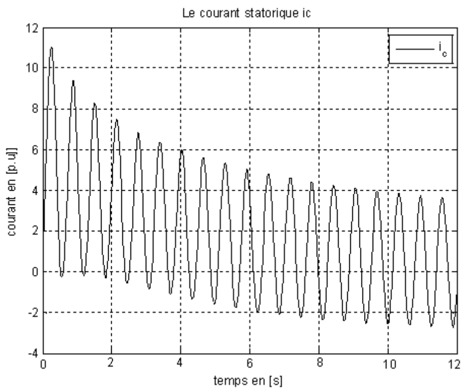
Figure : 7-3 Courant de phase statorique i_c .
