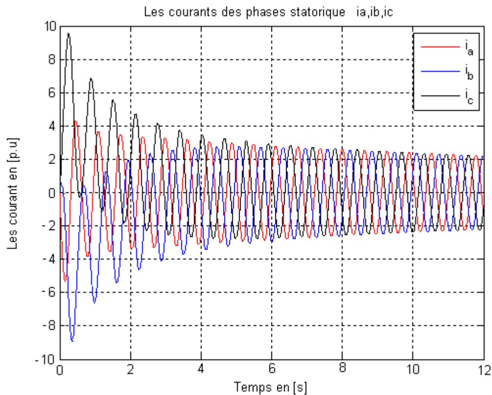
Figure : 7- 4- Les Courants des phases statorique i_a , i_b , i_c .
