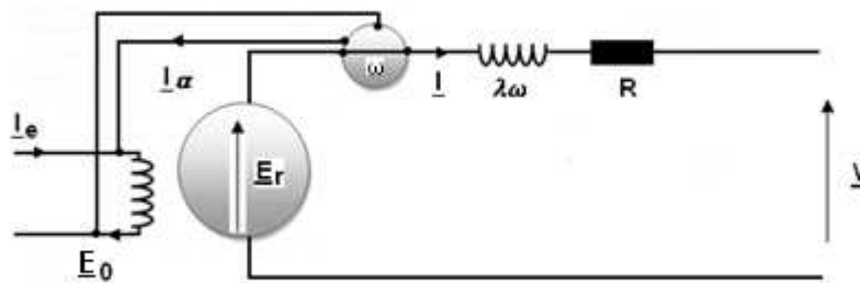
Figure4-5 : Schéma équivalent à un enroulement d'une génératrice synchrone.
