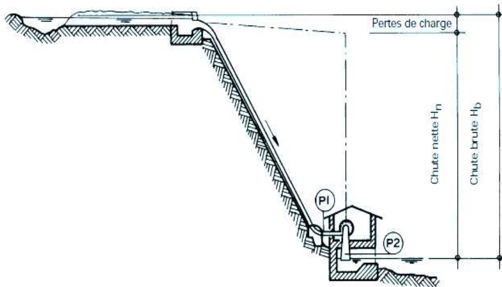
Figure. 1 -2 : Hauteur de chute brute et nette d'une microcentrale à conduite forcée.
