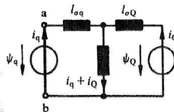
Figure 6-3 : Schéma équivalent pour les flux dans l'axe transversal [cf.1].
