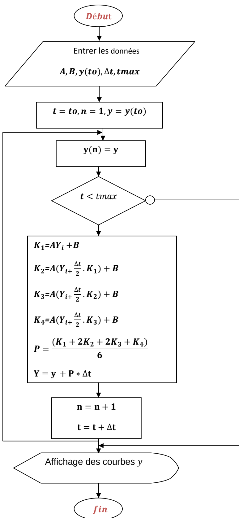
Figure : 6-6 l'Organigramme de la méthode RUNGE –KUTTA
